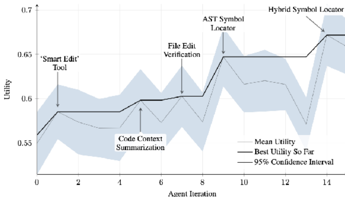
图 2：跨迭代的性能表现。关键改进用其相应的工具或智能体修改进行标注。（由 Maxime Robeyns、Martin Szummer、Laurence Aitchison 提供）
