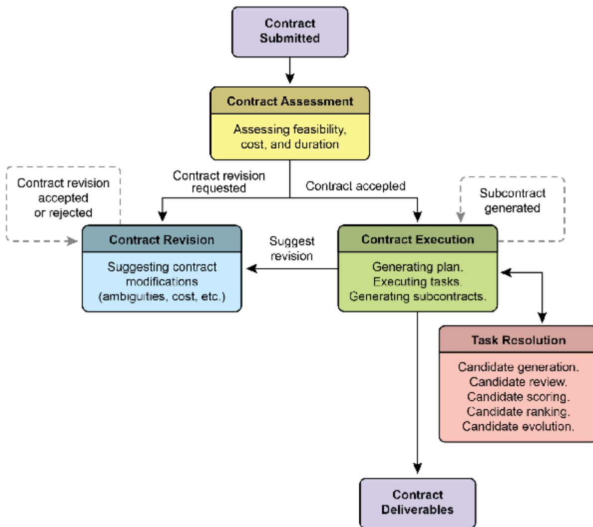
图 2：智能体之间的合约执行示例
